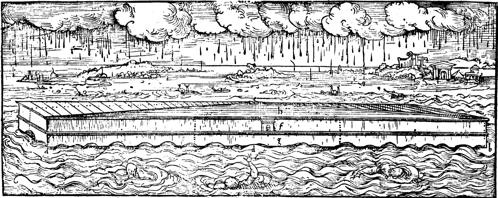
a b Longitudo 300 cubitorum. c Latitudo 50 cubitorum. d e Altitudo 30 cubitorum. f Ostium. g h i Fenestra longitudinis vnus cubit. Tristega, siue tabularia tria.
